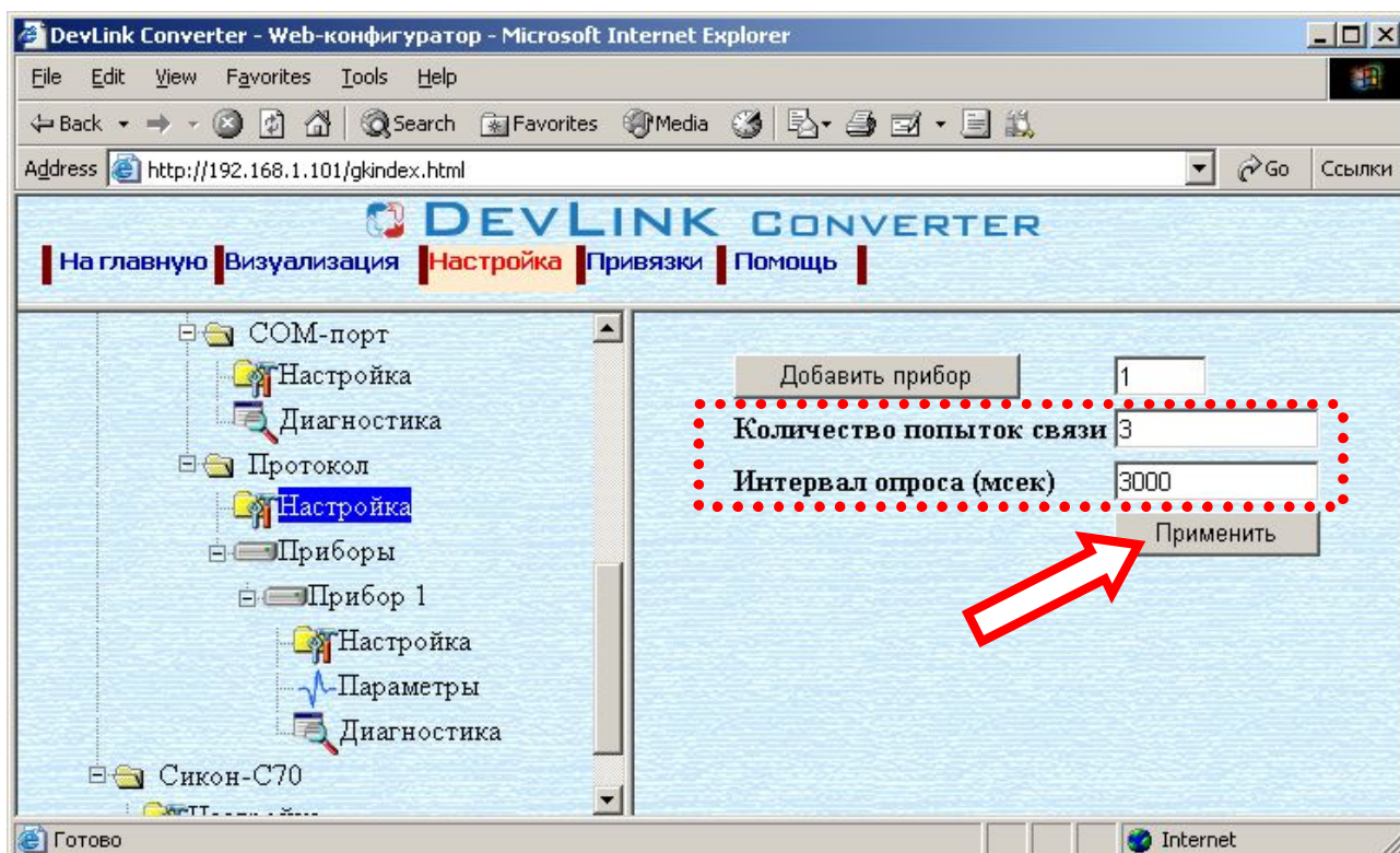
Рисунок 3.9 – Настройка протокола
